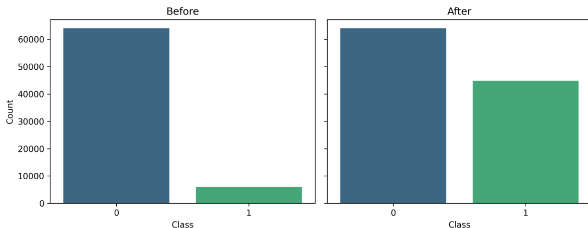
Figura 10 – Distribuição ajustada com SMOTE..
