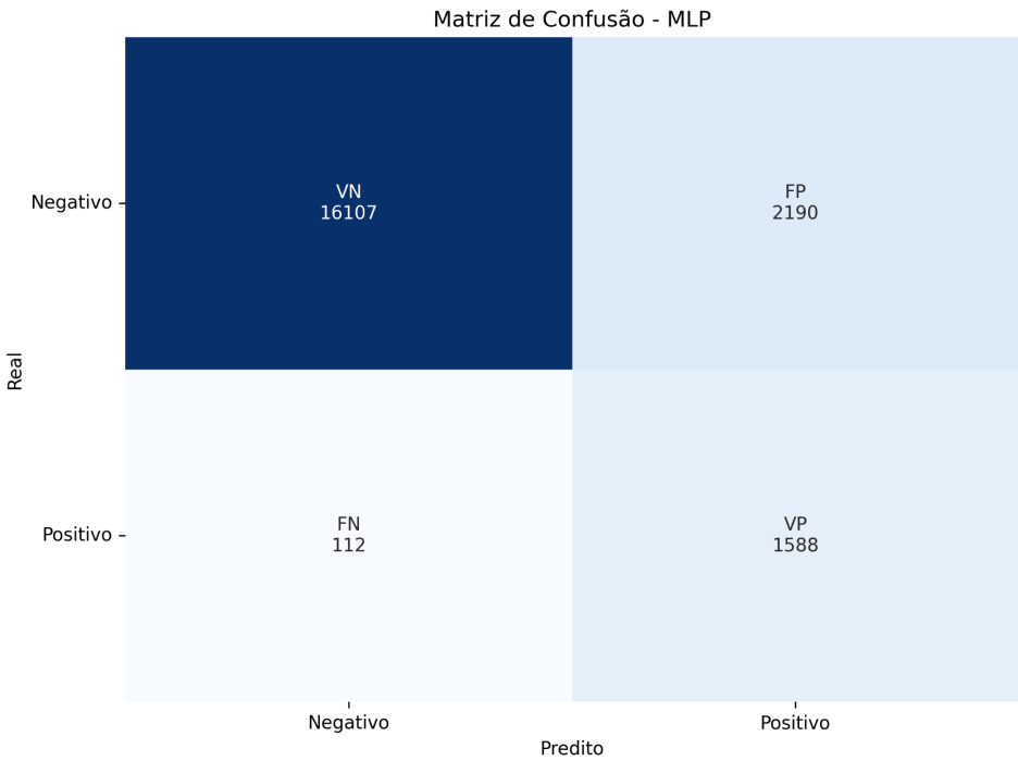
Figura 12 – Matriz de Confusão MLP..
