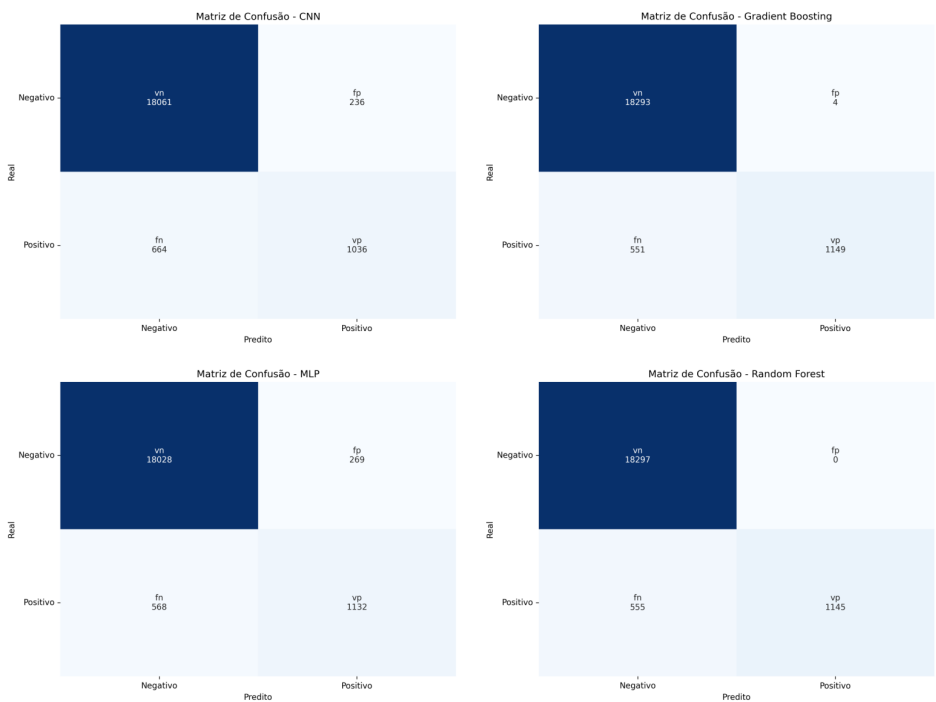
Figura 11 – Matriz de confusão..
