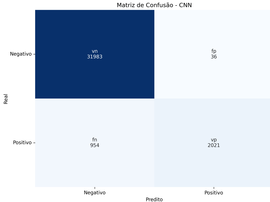
Figura 13 – Matriz de Confusão CNN..
