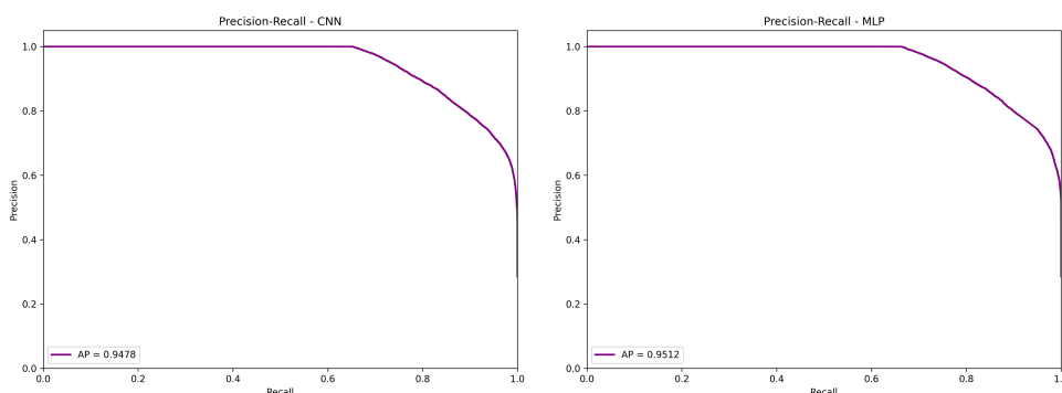
Figura 14 – Resultados: Curva Precision Recall..
